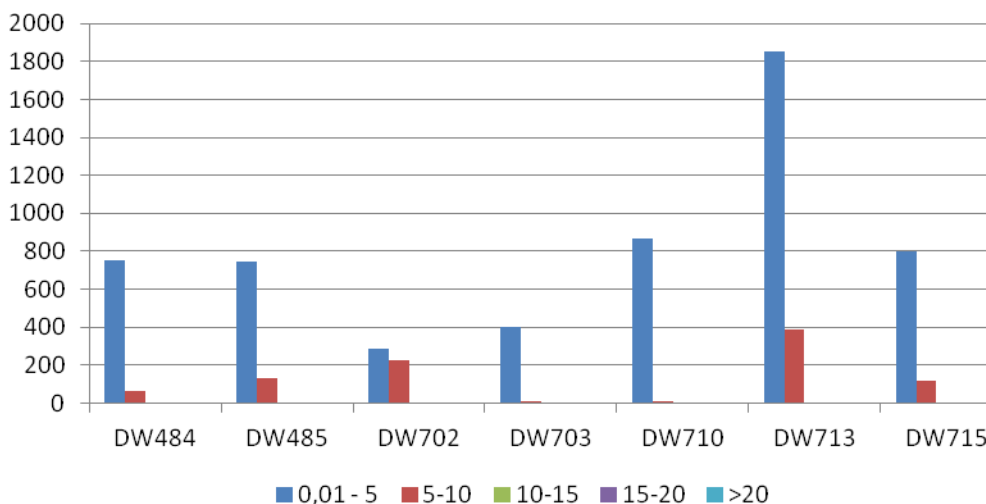
Rysunek 7 Liczba osób narażonych na przekroczenia wskaźnika L_N w otoczeniu odcinków dróg wojewódzkich administrowanych przez Zarząd Dróg Wojewódzkich w Łodzi
