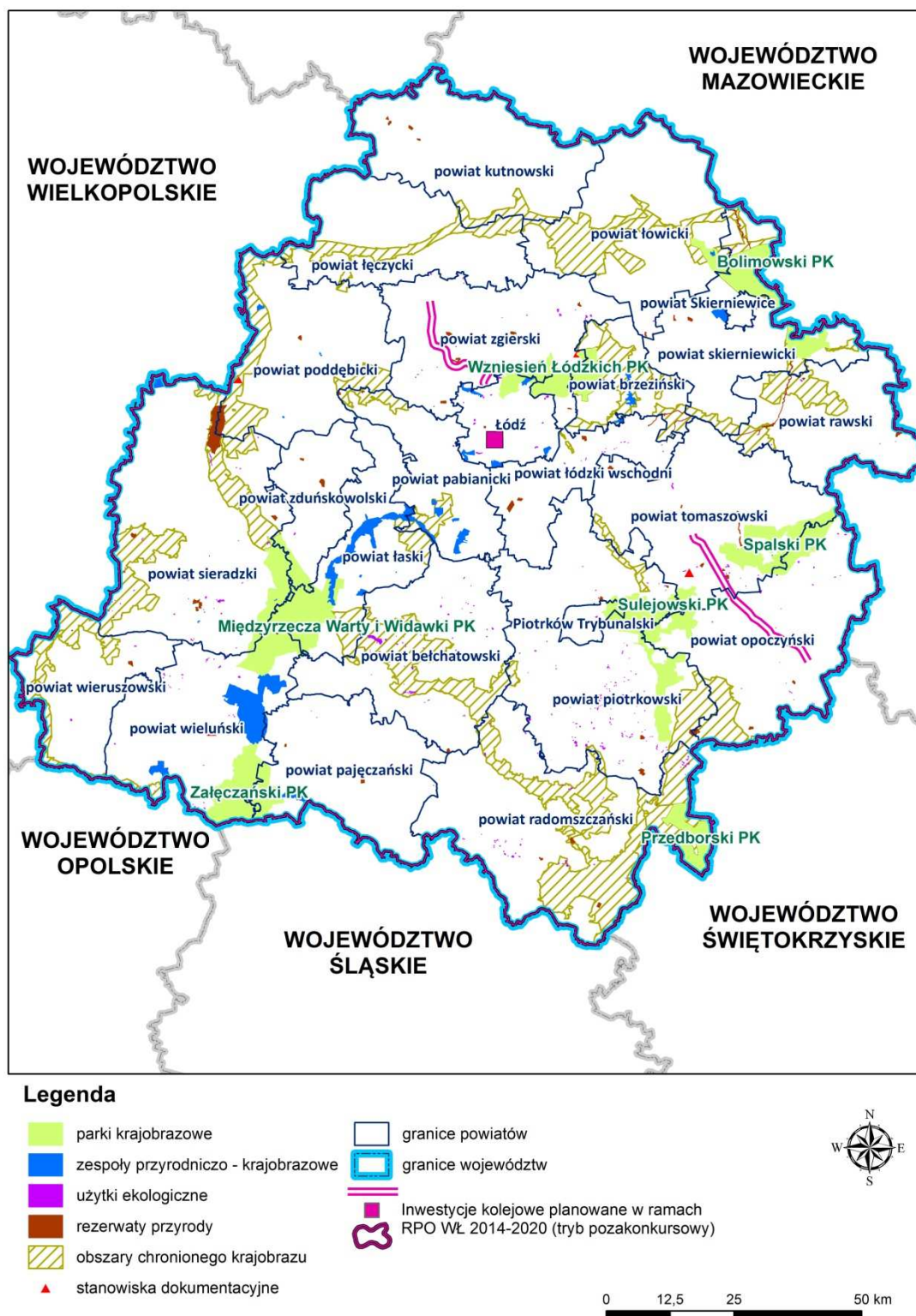
Rysunek 19 Planowane inwestycje kolejowe na tle obszarów chronionych (z wyłączeniem obszarów Natura 2000) 90 .
